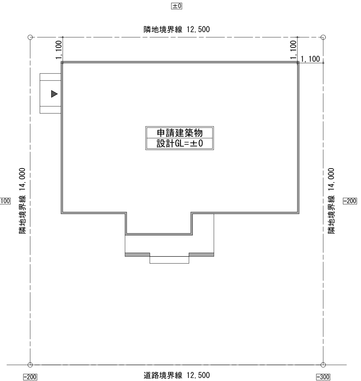
建物配置図 S=1/100
