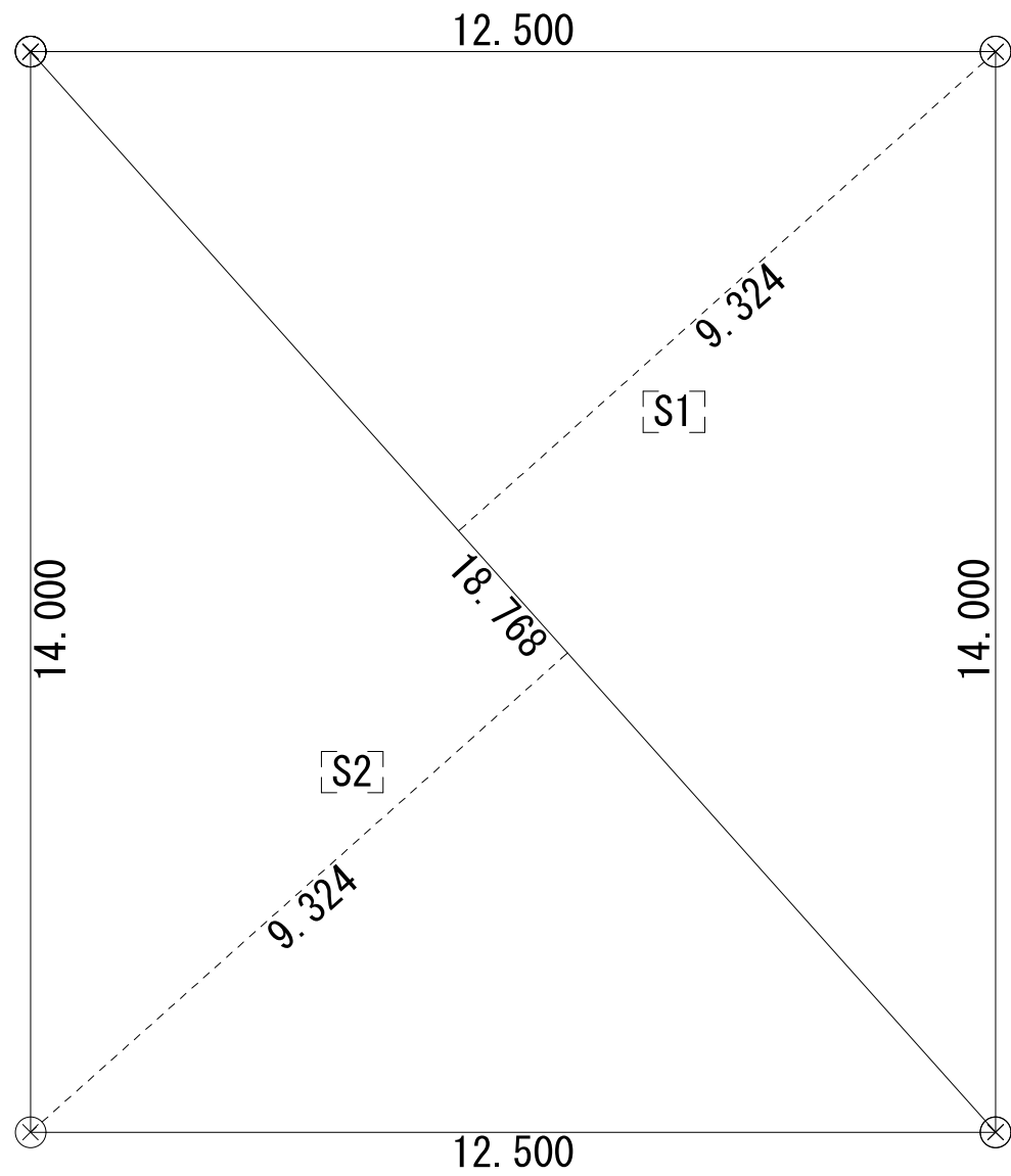
敷地求積図 S=1/100
