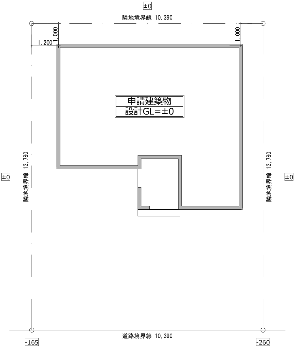
建物配置図 S=1/100
