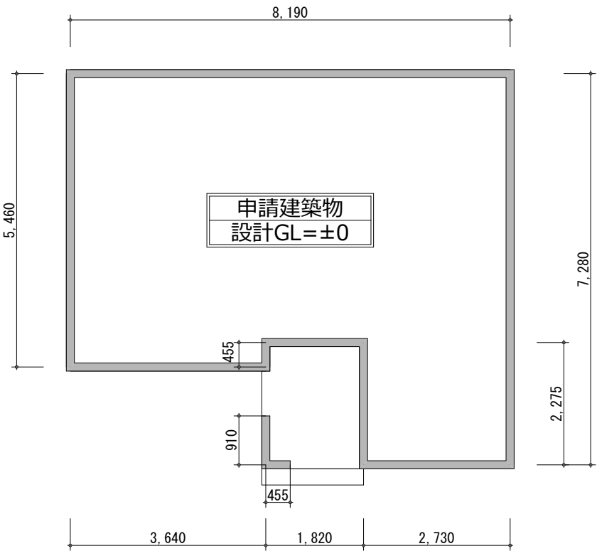
建物寸法 S=1/100
