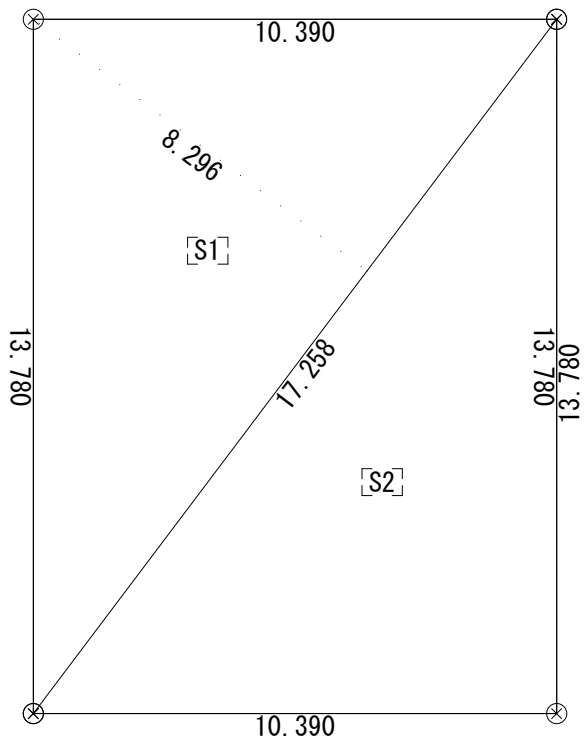
敷地求積図 S=1/150
